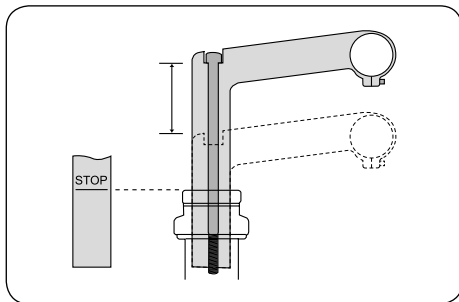
Höhenverstellung möglich
