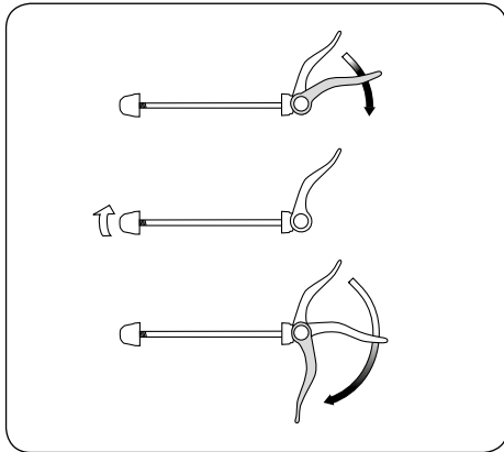
Instelmoer losdraaien
