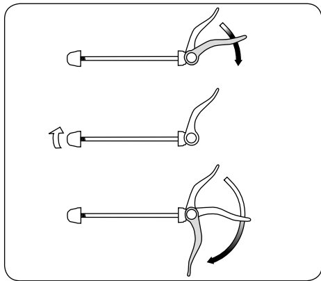
Alojar la tuerca de reglaje
