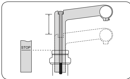
Altura regulable
