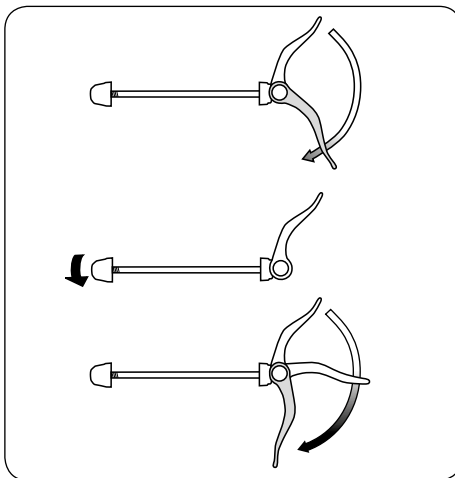
Serraggio del dado di regolazione
